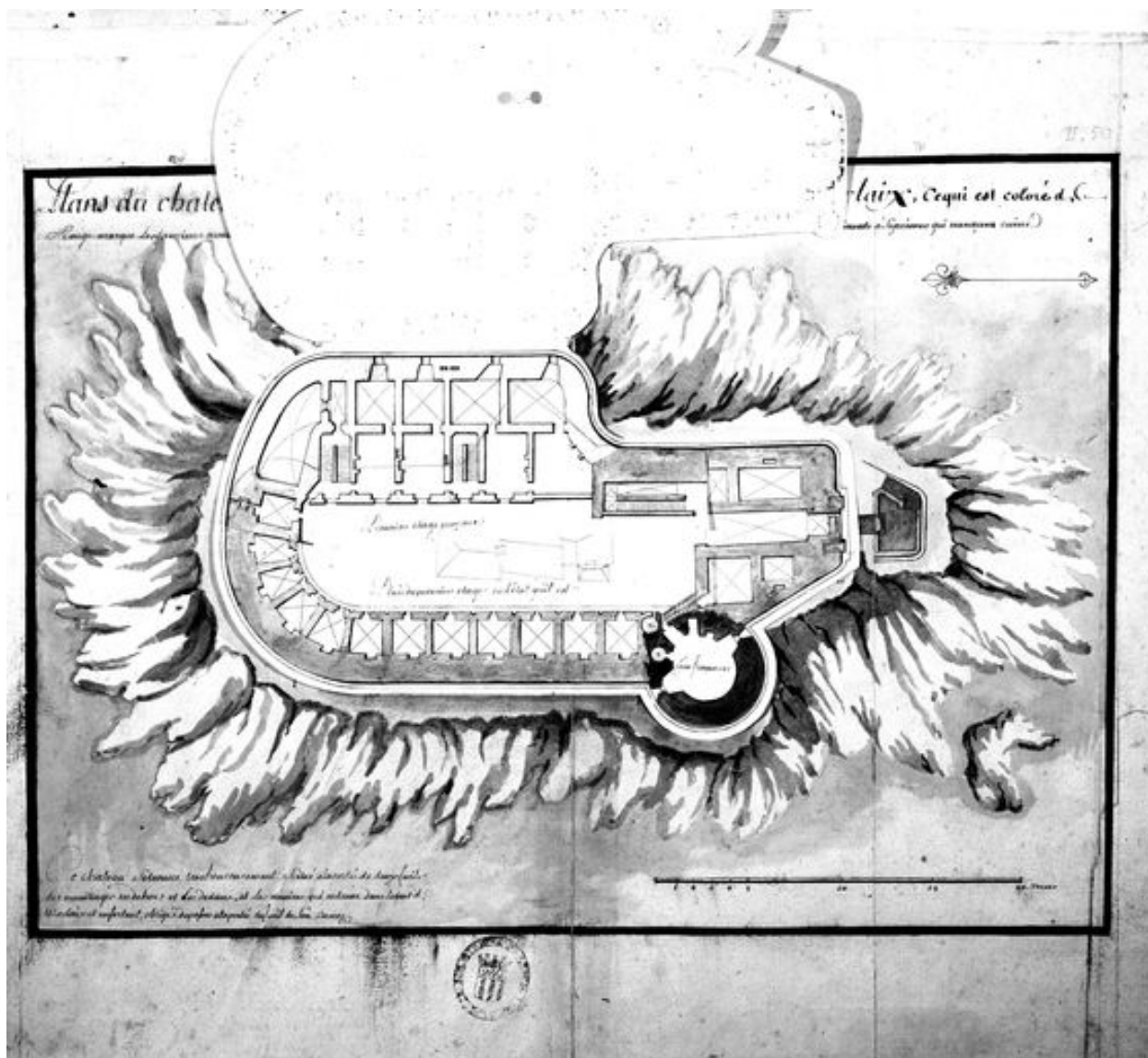
Plan du 1er étage : projet d'agrandissement, sans date
