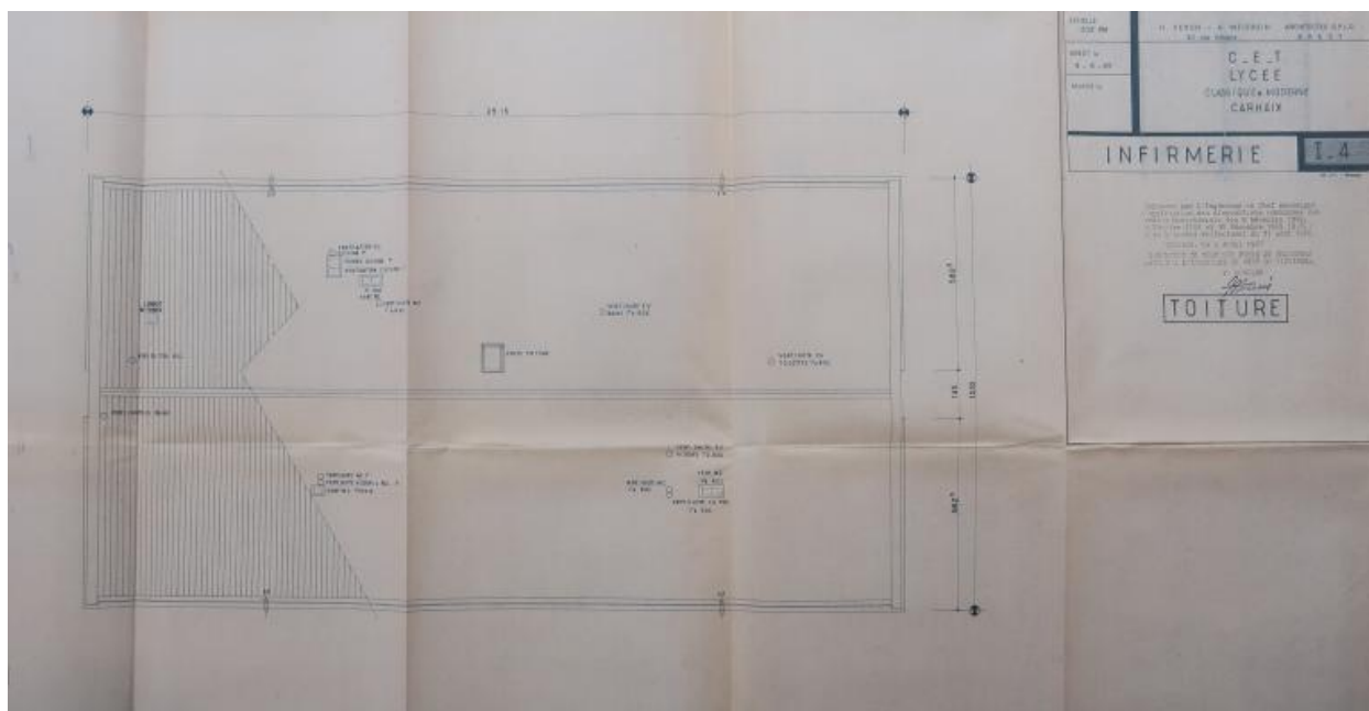
Plan de la toiture, H. Péron et A. Weisbein, architectes, 08/06/1965.
