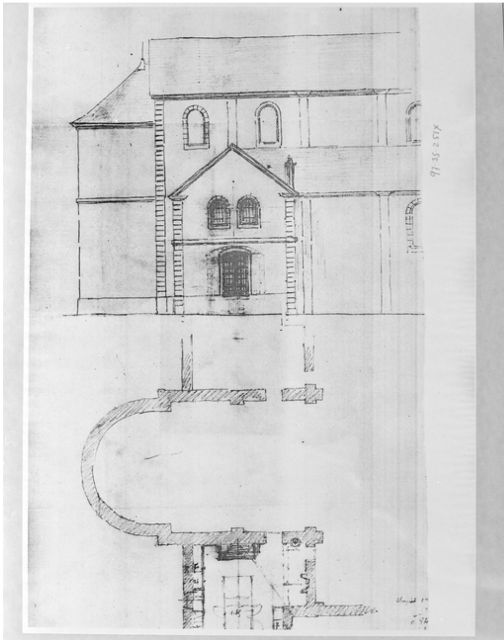
Plan du choeur et de la sacristie, élévation de la sacristie.
