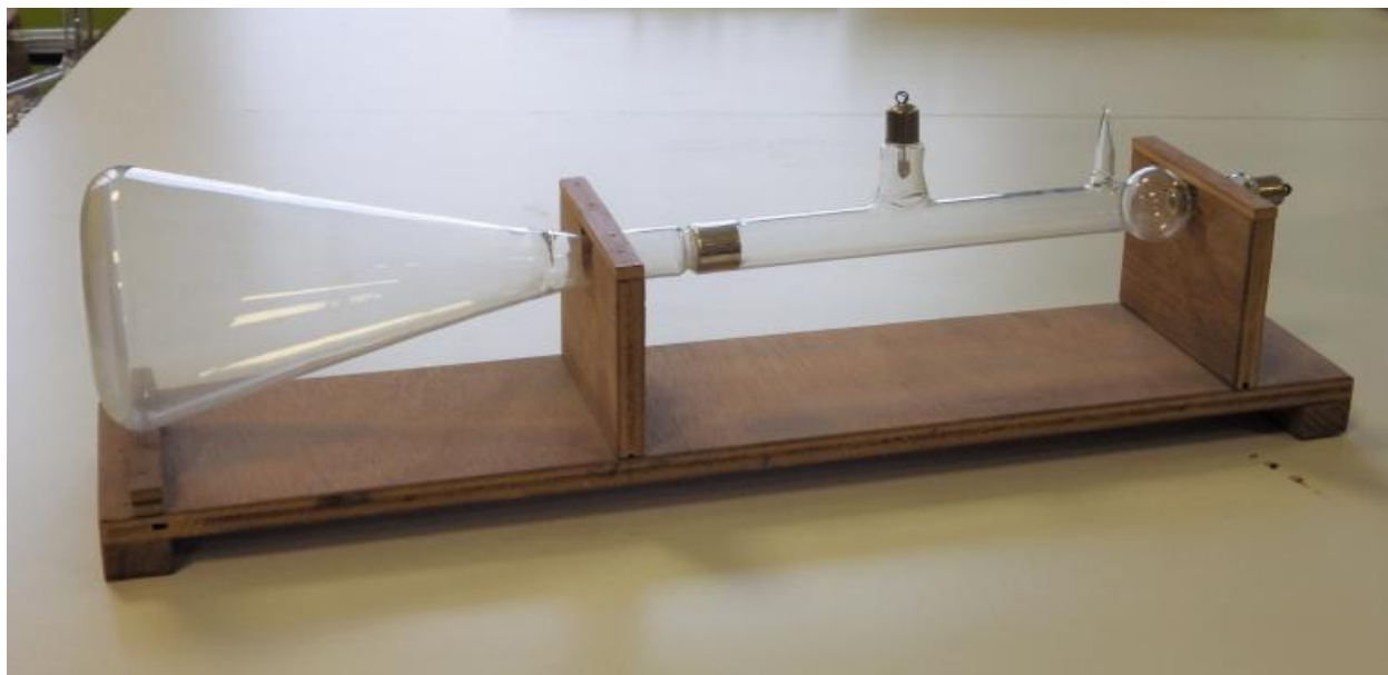
Tube à vide de Braun - Electricité dynamique (Non signé)
