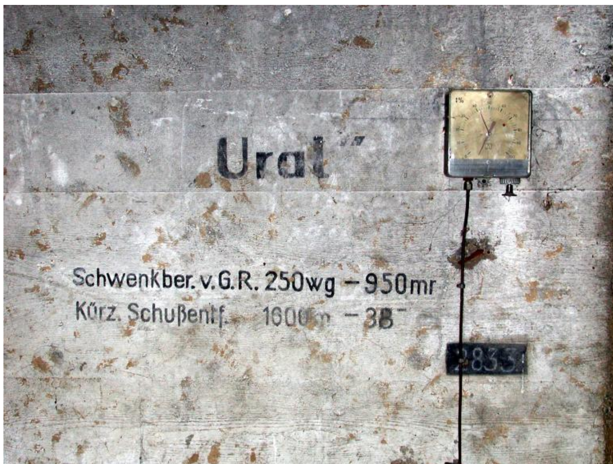
Vue intérieure de l'un des bunkers de type 669 (quatrième casemate) : Ural (nom du bunker) et instructions de tir (état en 2003)
