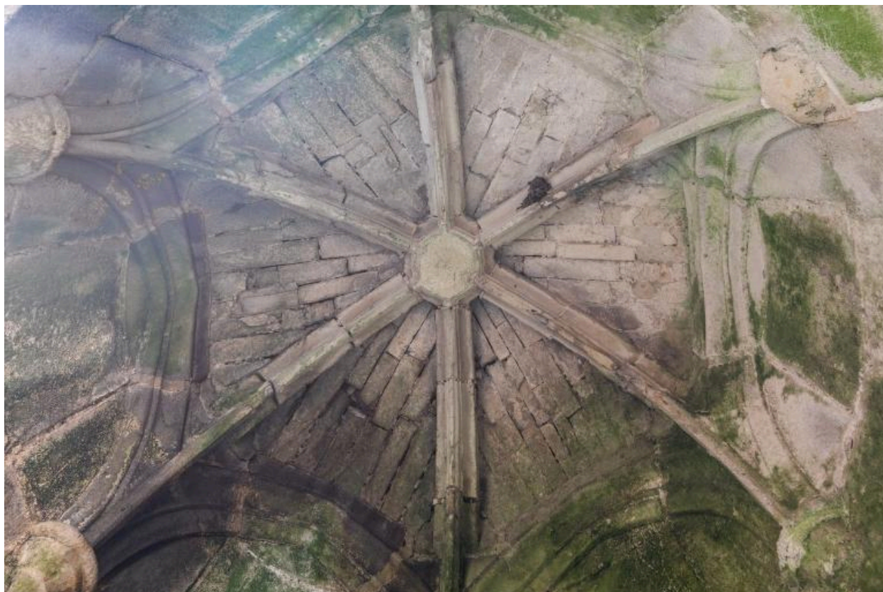
Vue de la voûte de la tourelle sud.
