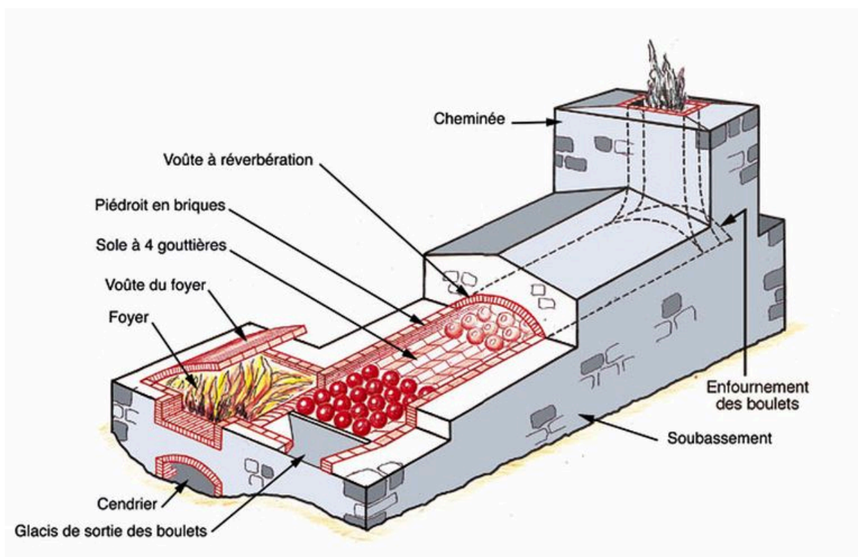
Vue axonométrique d'un four à boulets de type Meusnier (1793)
