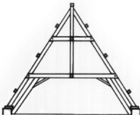
Coupe transversale (arbalétrier en 3 pièces)
