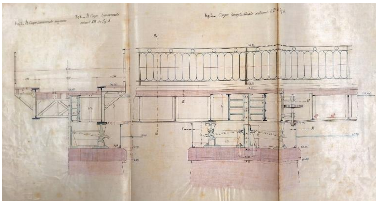
Coupe transversale du mécanisme du mouvement de rotation (28 mai 1891)
