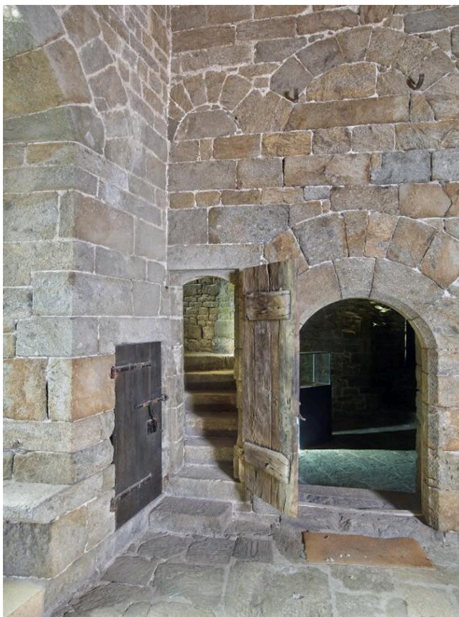
Vue intérieure de la tour Solidor : rez-de-chaussée, pièce intermédiaire, détail du mur de refend ouest. Au centre, la porte des latrines (en niveau intermédiaire) ; à gauche, placard mural (ancienne poterne) ; à droite, la porte de la tour ouest
