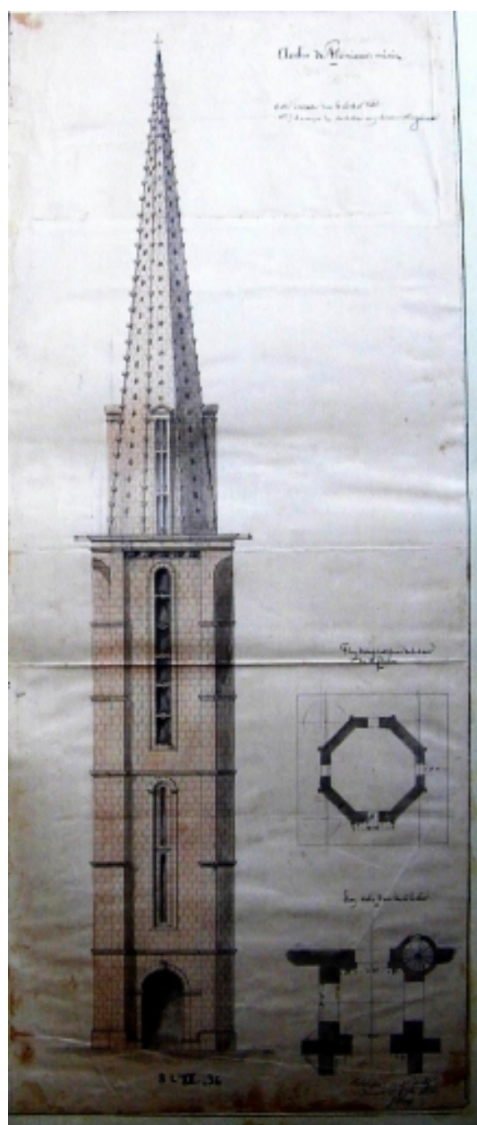
Le clocher. Relevé par Joseph Bigot, 1855 (A. E. Quimper, 8 L XII, 36)
