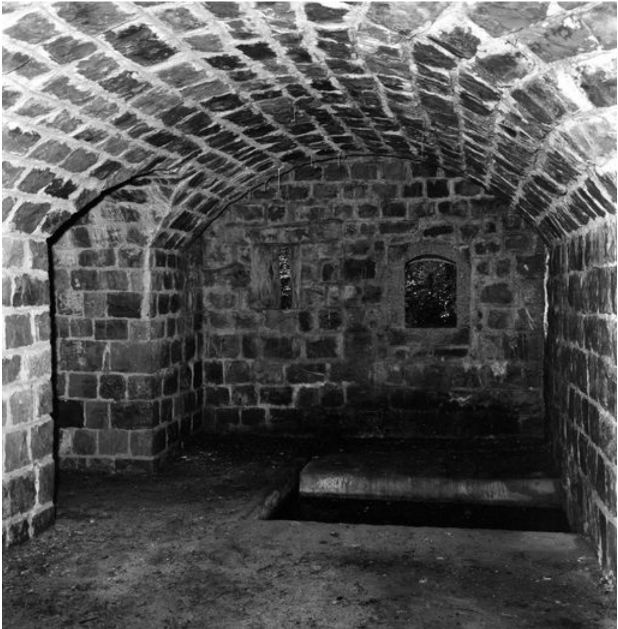
Vue du réduit de Landaoudec en 1969 : caponnière, chambre de tir. A droite : créneau du canon-révolver, à gauche : créneau de fusillade
