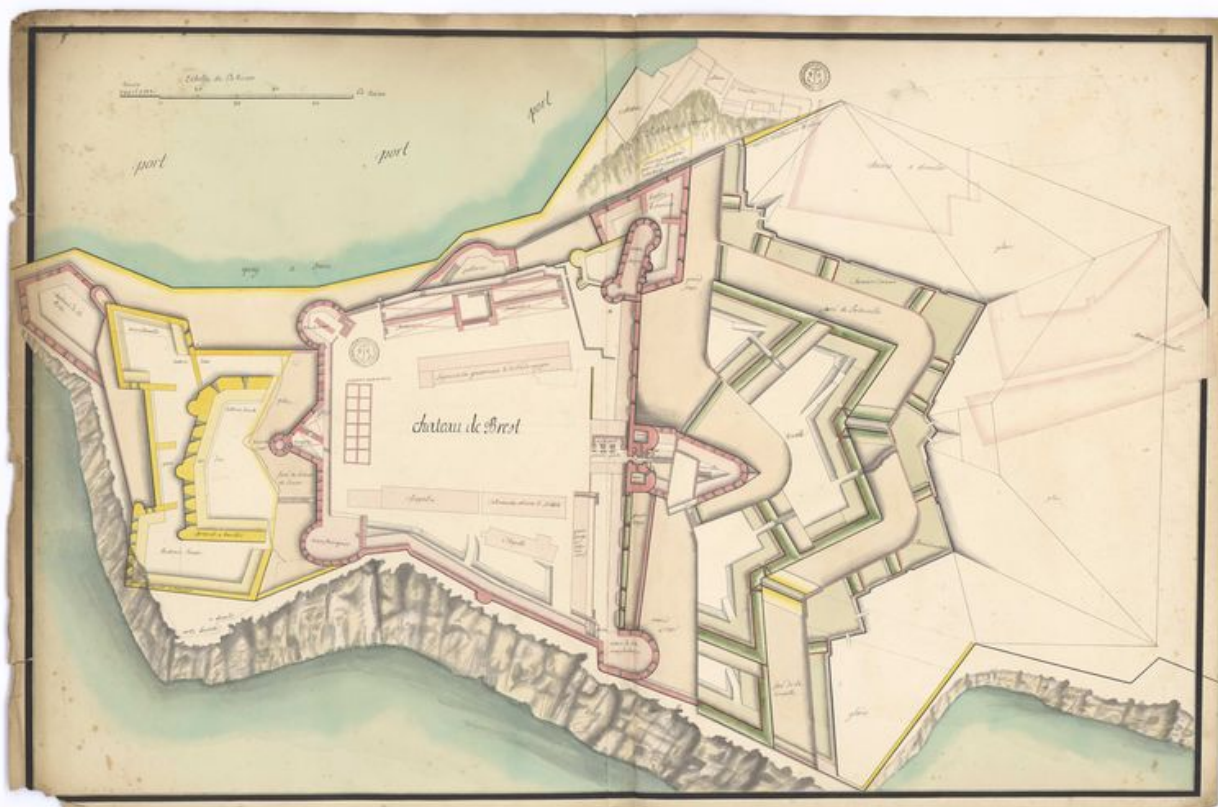
Plan du château de Brest, projet de transformation des batteries du Parc-au-Duc. 1er quart 18e siècle
