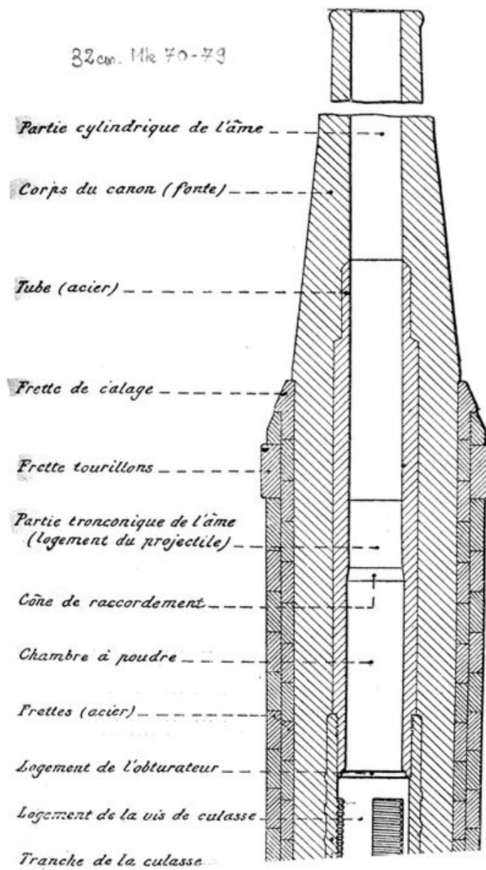
Coupe d'un canon de 32 cm modèle 1870-1879 (armement de la batterie extérieure du Portzic sur affût M modèle 1876-T-83 PA)
