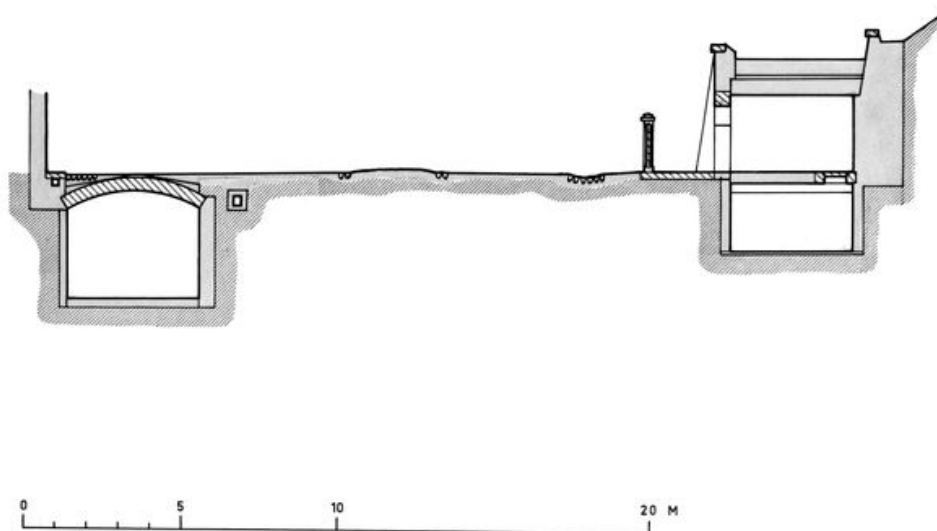
COUPE SUIVANT O.P.
