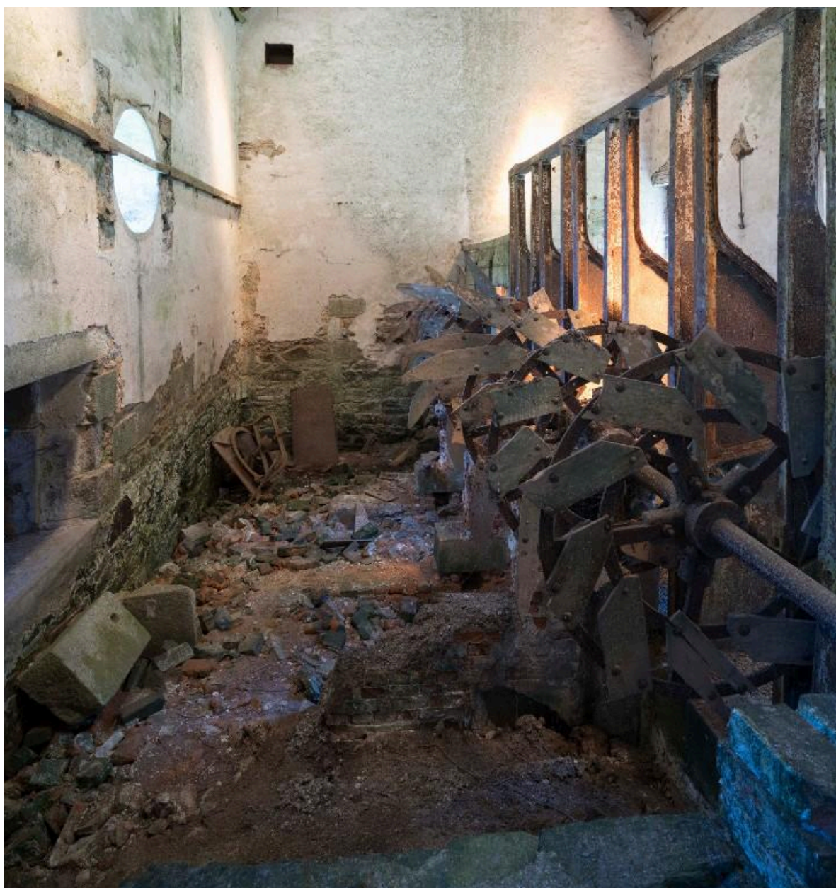
Bâtiment principal. Salle 3, dite salle d'espilage. Mécanisme de teillage et fosse à étoupe et à chènevotte
