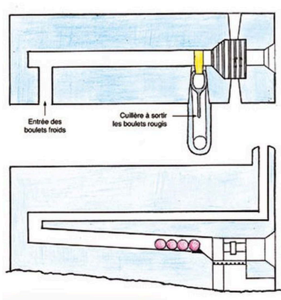
Coupes du four du fort Cézon à Brest (1810)
