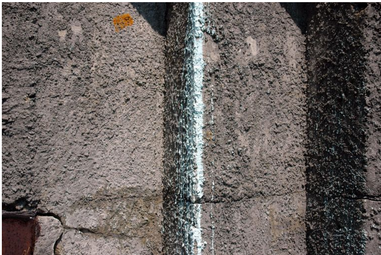
Vue de l'un des deux bunkers - casemates de type 671 (état en 2005). Le traitement du béton participait du camouflage du bunker
