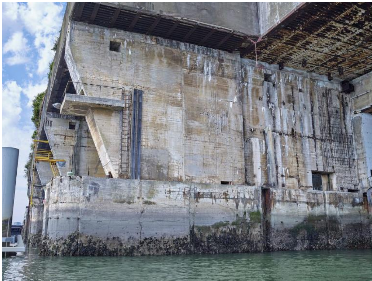
Vue de l'entrée de l'alvéole F (n° 15 et 16) : contrefort du mur latéral
