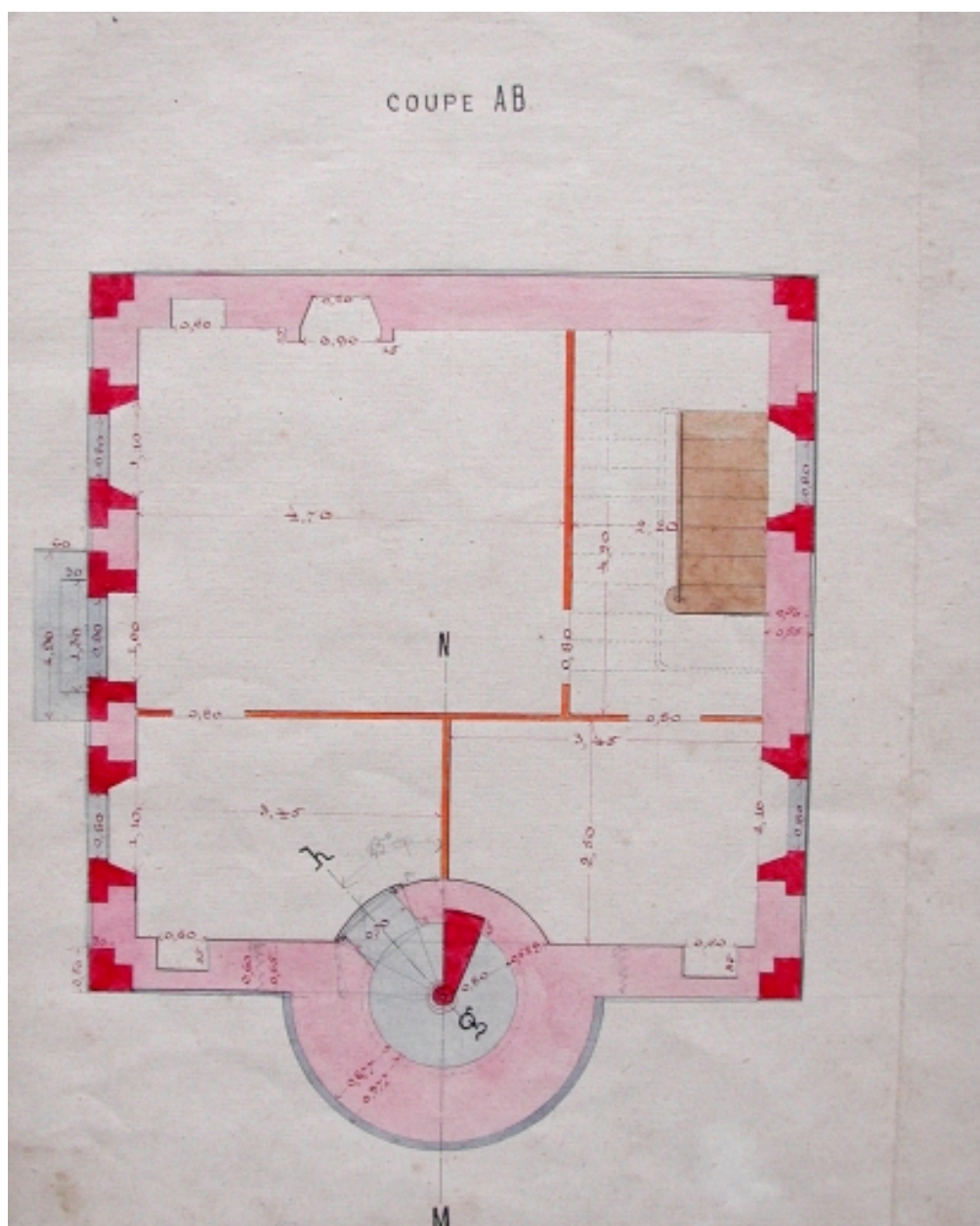
Transformation du feu : dessin en coupe, 1882 (AD 22)
