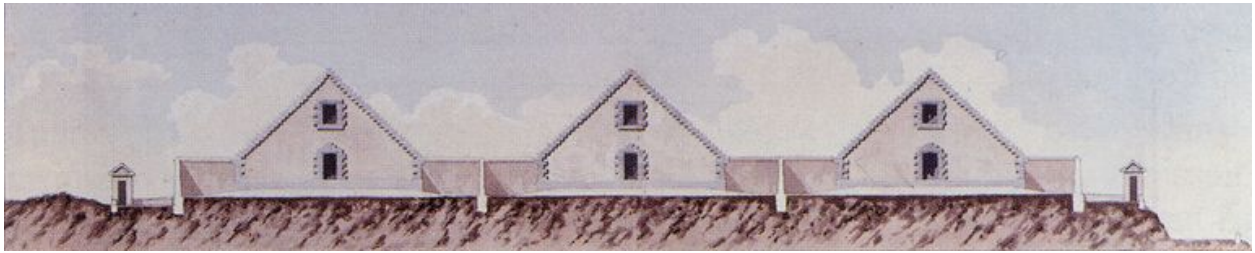
Elévation des trois magasins à poudre dits "poudrières maritimes" de l'île des Morts, Travaux Maritimes, 1813
