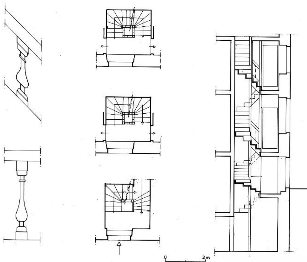
Maison, escalier : coupe, plan et détails des balustres (état en 1994)
