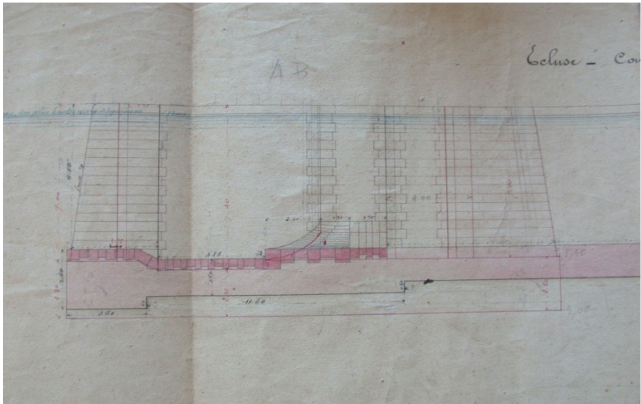
Dessin : coupe transversale d'un vantail de la 1ère écluse, 1875 (AD 22)
