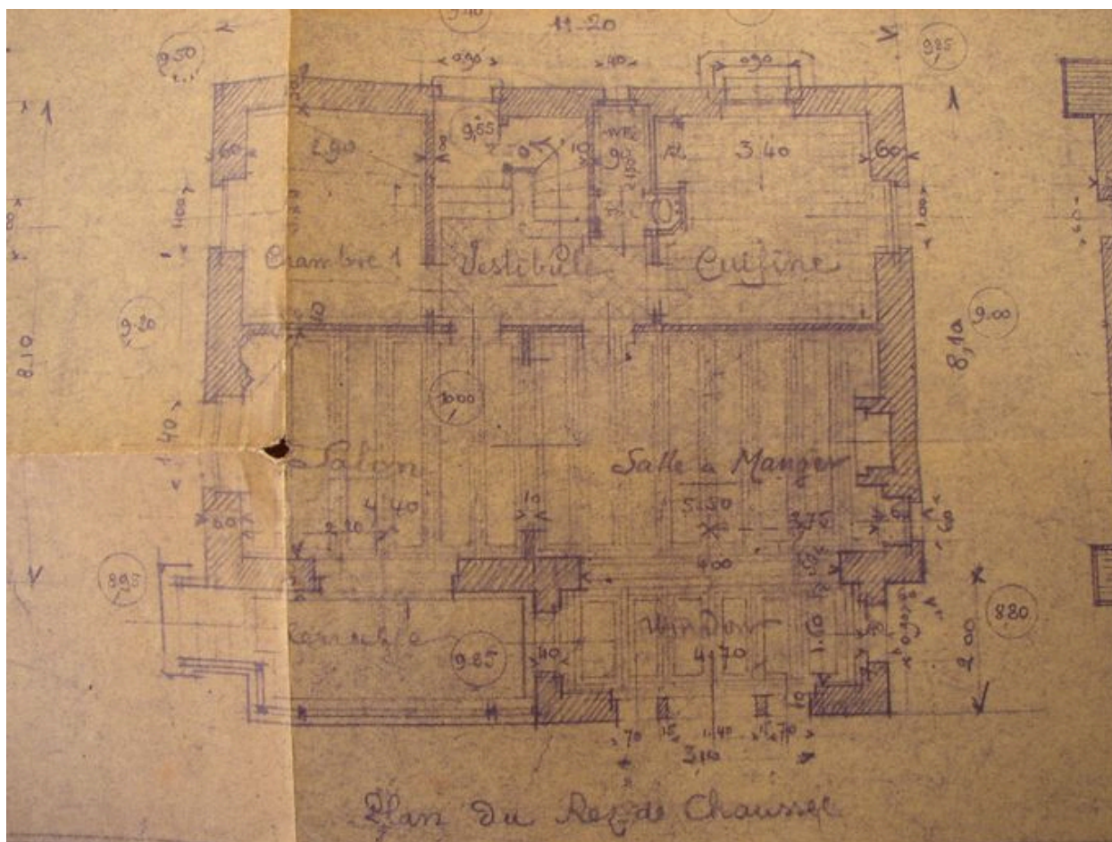
Plan du rez-de-chaussée de la villa Les Fuchsias
